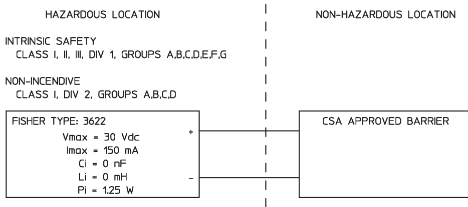
Рис. 31. Схема контуров для Fisher 3622 по CSA
