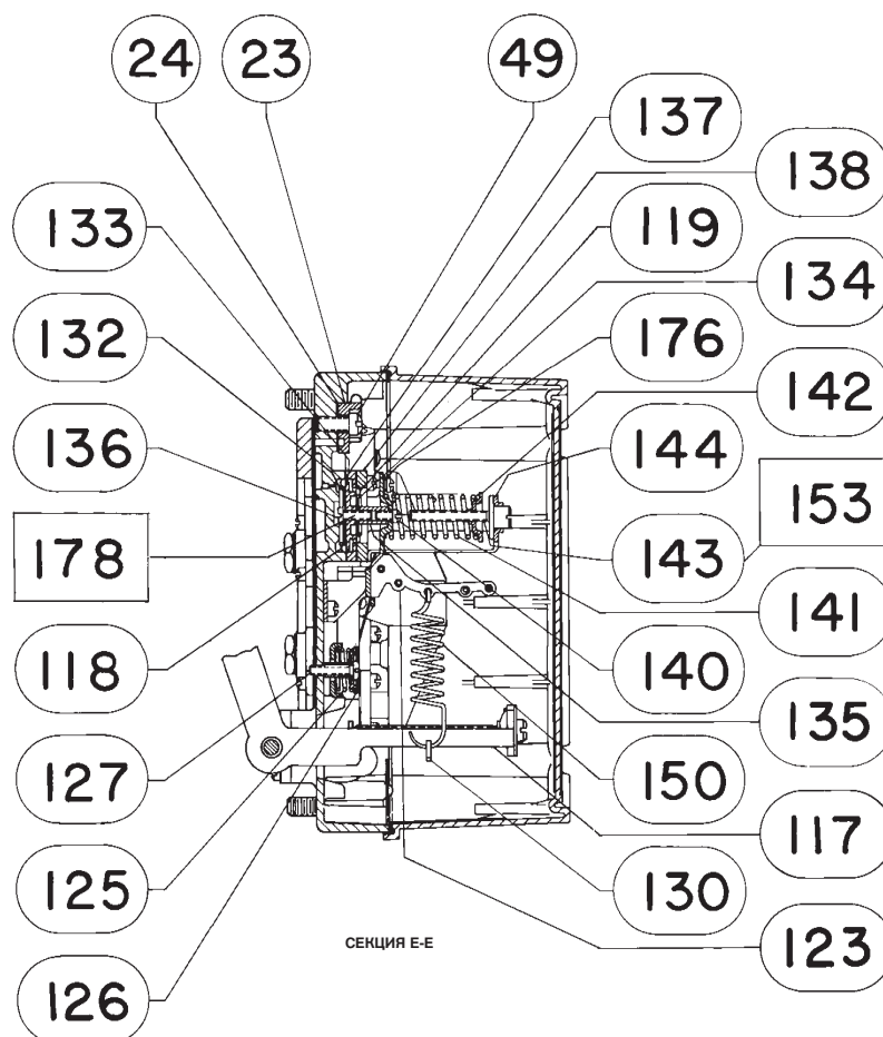
Рис. 25. Позиционеры в сборе (продолжение)
