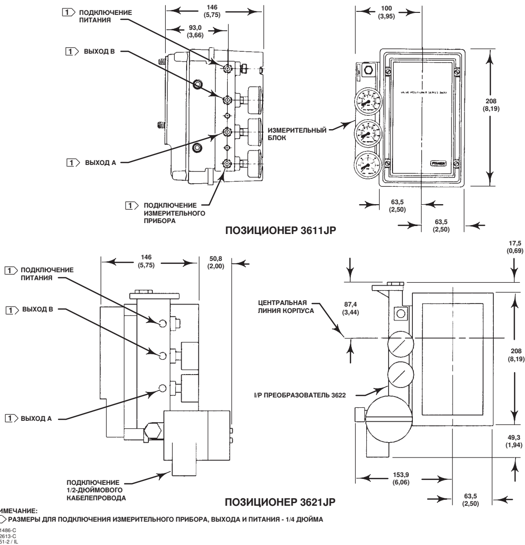
Рис. 8. Размеры и соединения при типовом монтаже (продолжение)
