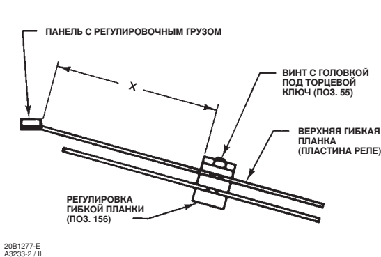
Рис. 14. Регулировка коэффициента усиления вспомогательного контура
