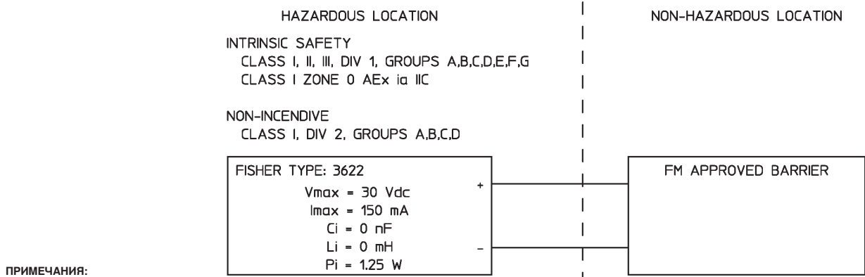
Рис. 33. Схема контуров для Fisher 3622 по FM
