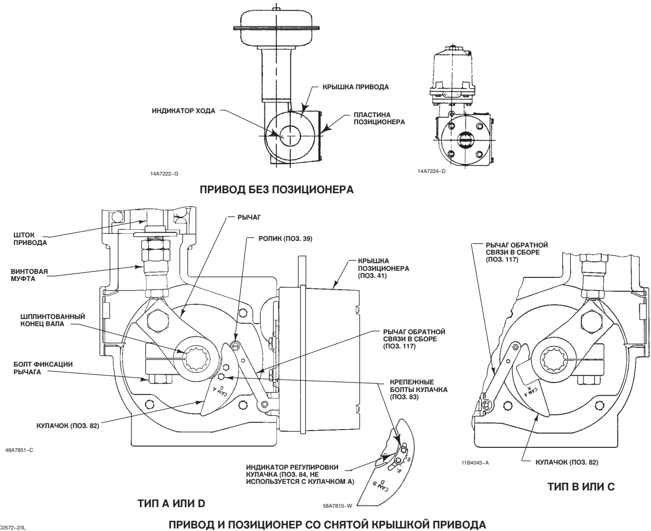
Рис. 3. Монтаж позиционеров Fisher 3610J и 3620J на поворотных приводах
