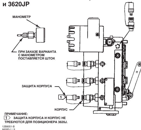
Рис. 10. Подключение системы диагностики FlowScanner для позиционеров Fisher 3621J и 3620JP
