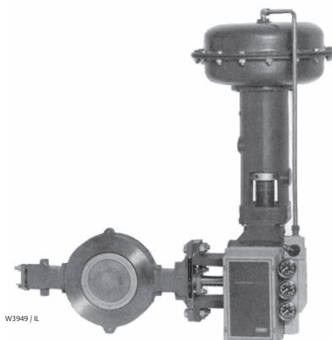
ПОЗИЦИОНЕР 3610J И БАЙПАСНЫЙ КЛАПАН С ПРИВОДОМ FISHER 1052 И ПОВОРОТНЫМ КЛАПАНОМ С ЭКСЦЕНТРИКОВЫМ ДИСКОМ
