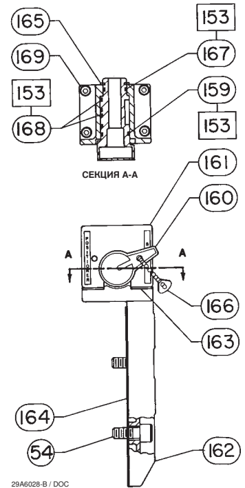
БАЙПАСНЫЙ КЛАПАН В СБОРЕ ДЛЯ ПОЗИЦИОНЕРОВ 3610J
