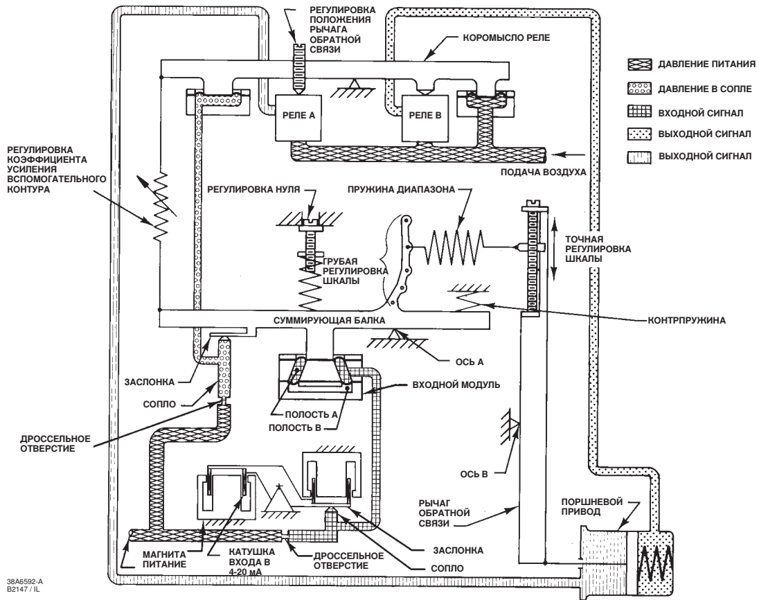
Рис. 24. Принципиальная схема позиционера Fisher 3621JP
