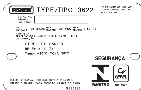
Рис. 35. Паспортная табличка соответствия стандартам INMETRO для позиционера Fisher 3622
