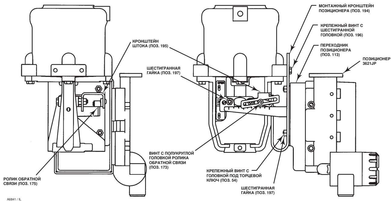
Рис. 5. Монтаж позиционеров Fisher 3611JP и 3621JP на приводе 585С
