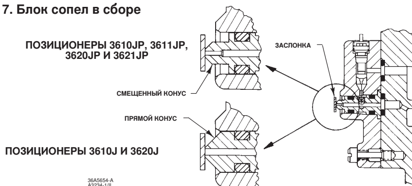
Рис. 7. Блок сопел в сборе
