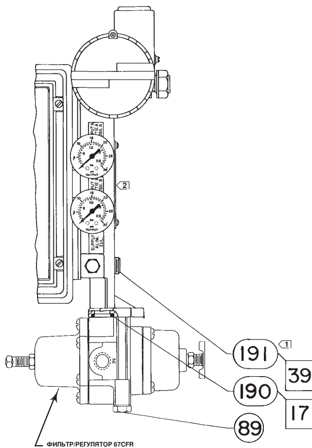
Рис. 27. Positioner Fisher 3620J со встроенным фильтром-регулятором
