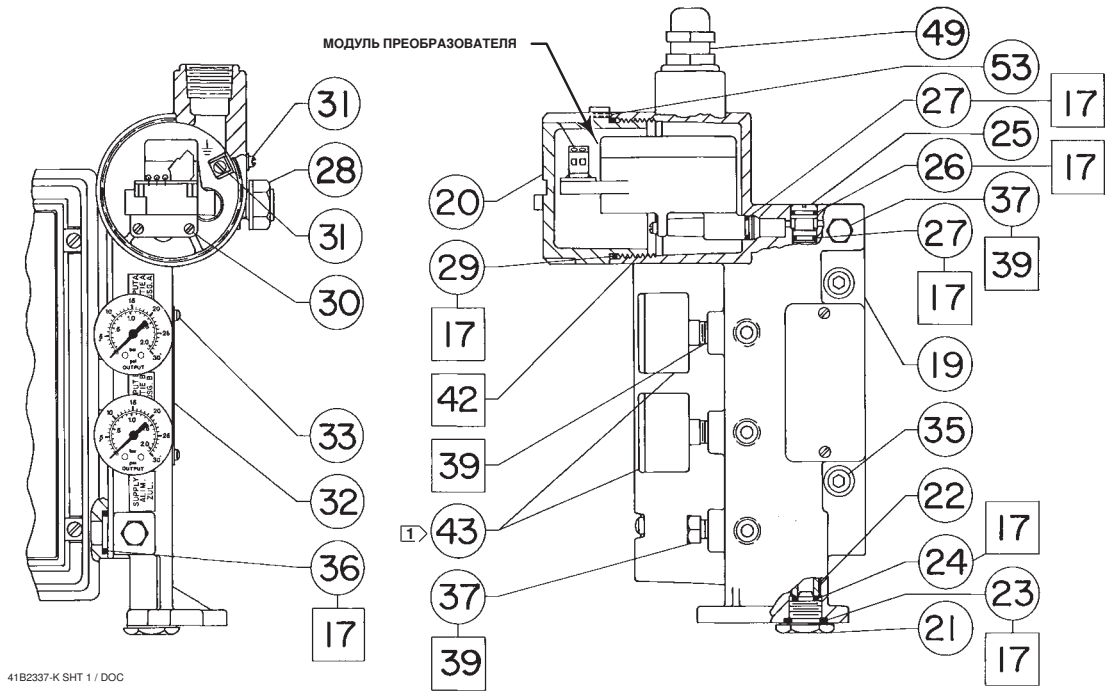
Рис. 30. Электропневматический преобразователь Fisher 3622
