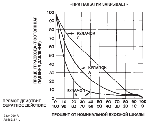
Рис. 18. Характеристики расхода для различных кулачков при использовании клапана с равнопроцентной характеристикой и действием при нажатии закрывает
