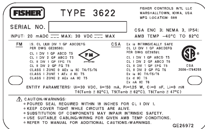
Рис. 32. Паспортная табличка соответствия стандартам CSA/FM для Fisher 3622
