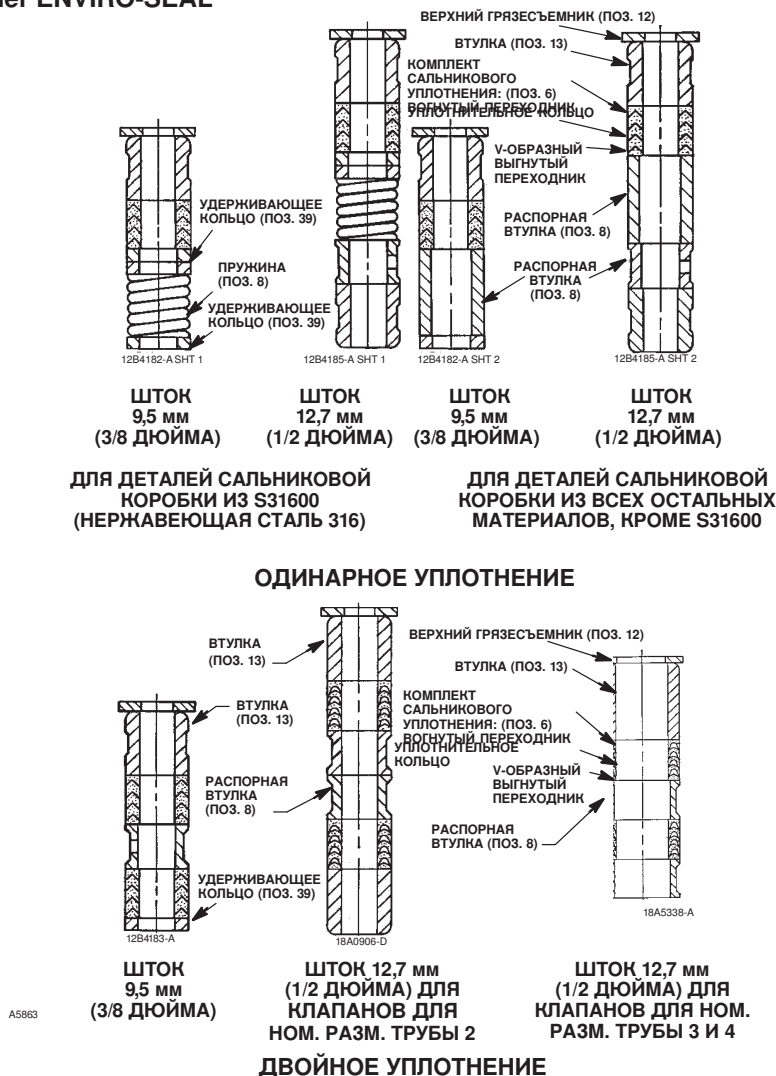
Рис. 6. Сальниковые уплотнения из ПТФЭ для применения в крышках сильфонных уплотнений Fisher ENVIRO-SEAL
