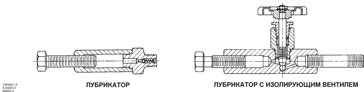
Рис. 2. Лубрикатор и лубрикатор/изолирующий вентиль (дополнительно)
