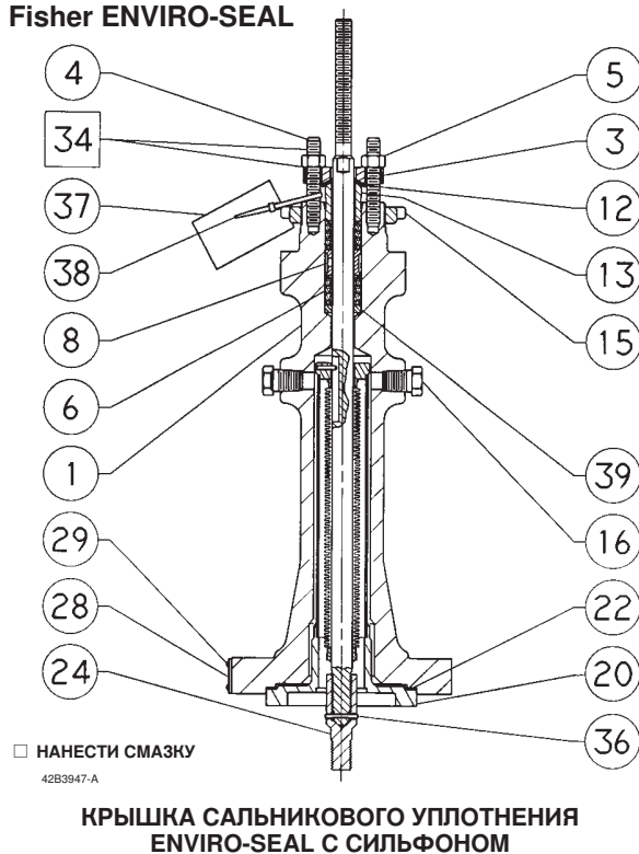
Рис. 15. Крышка сильфонного уплотнения Fisher ENVIRO-SEAL
