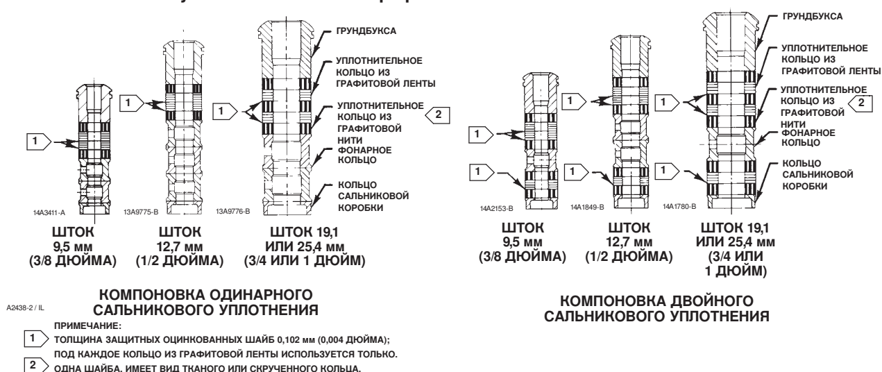
Рис. 5. Сальниковые уплотнения Fisher из графитовой ленты/нити
