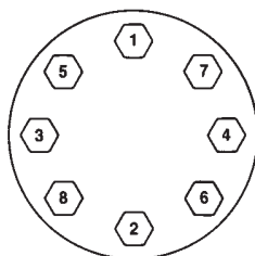
Рис. 8. Стандартная схема затяжки болтовых соединений
