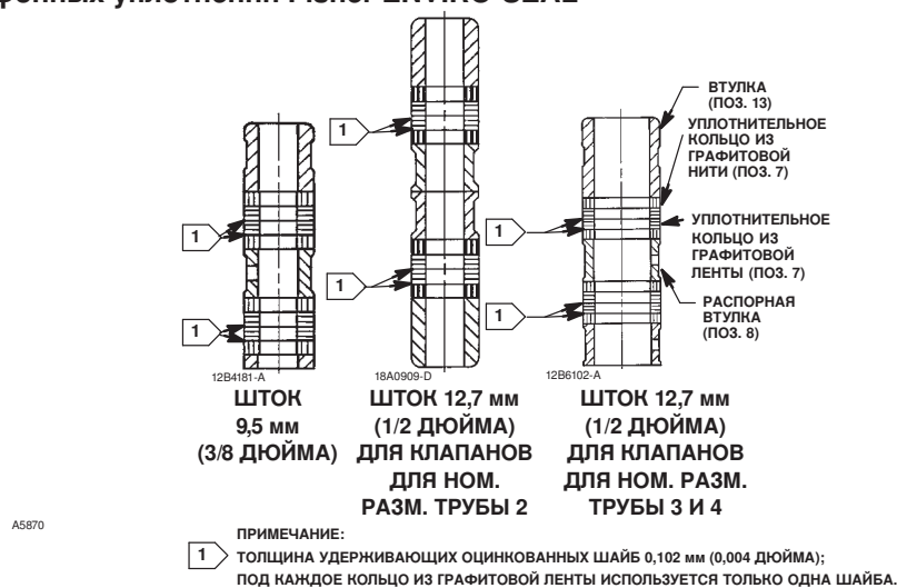
Рис. 7. Двойные сальниковые уплотнения из графитовой ленты/нити для применения в крышках сифонных уплотнений Fisher ENVIRO-SEAL
