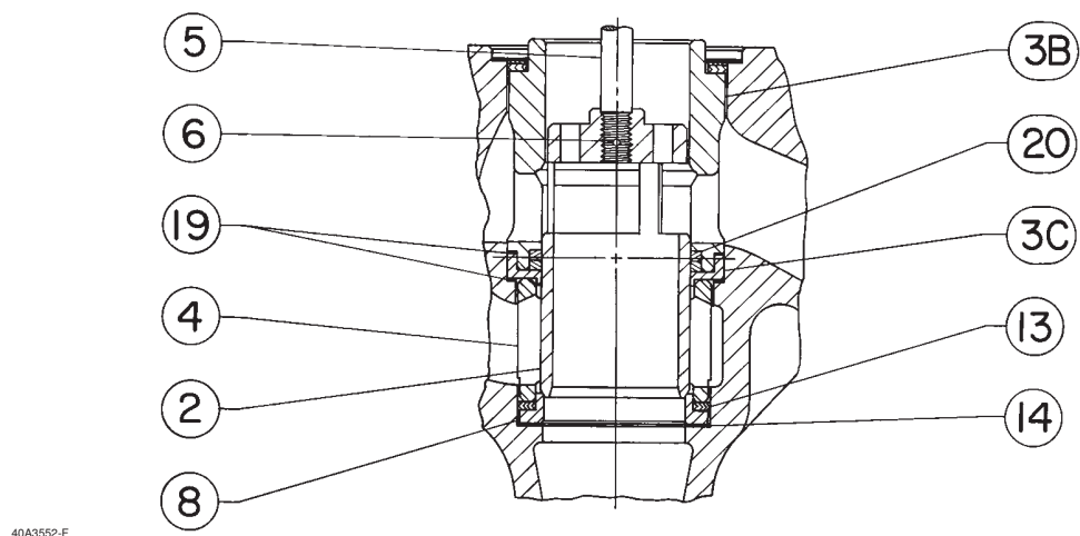
Рис. 11. Клапан Fisher YD (исполнение для высоких температур)
