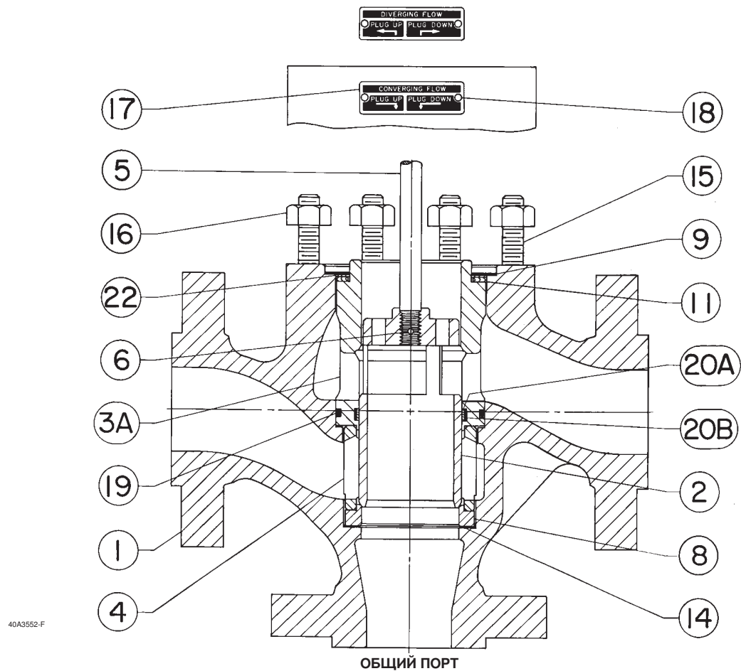
Рис. 10. Клапан Fisher YD (стандартное исполнение)
