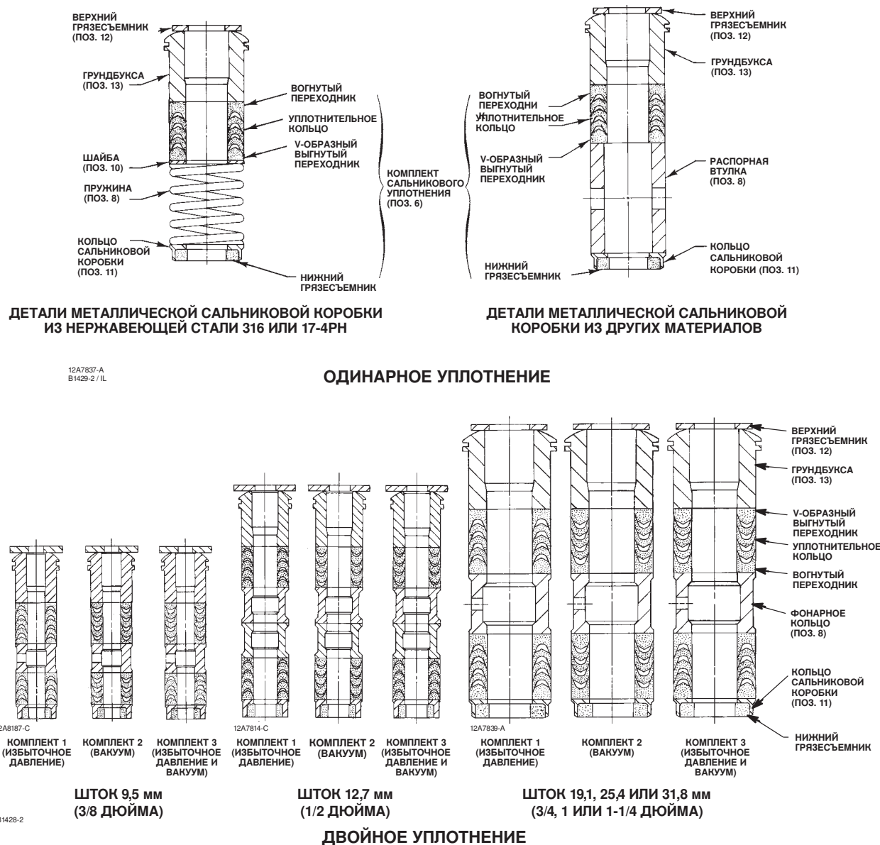
Рис. 3. Сальниковые уплотнения Fisher с V-образными кольцами из ПТФЭ
