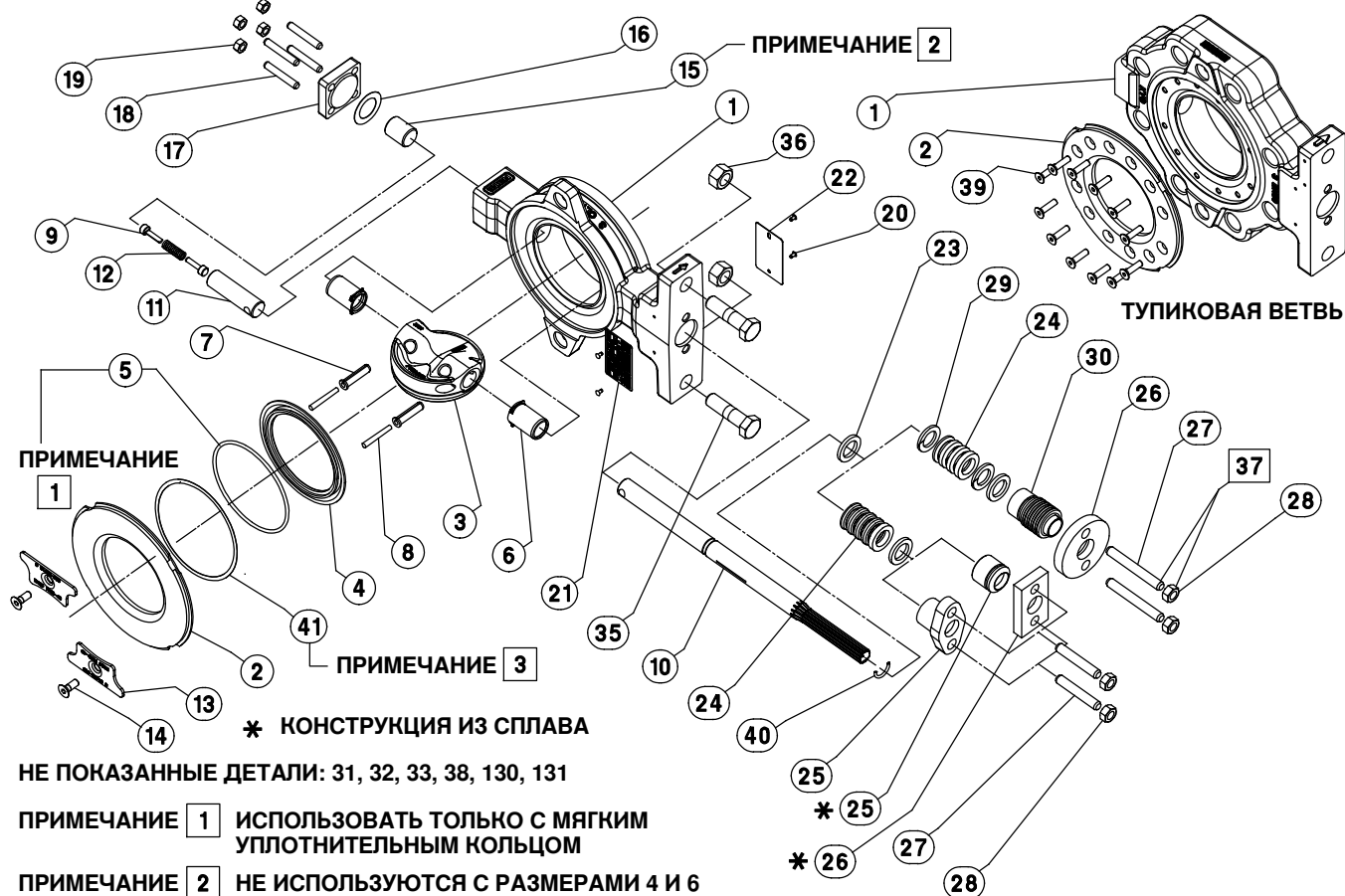
Рис. 11. Узел затвора Fisher Control-Disk
