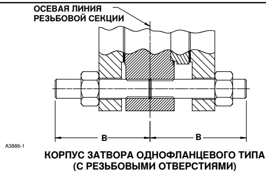
Рис. 3. Резьбовые шпильки для установки (также см. таблицу 5)
