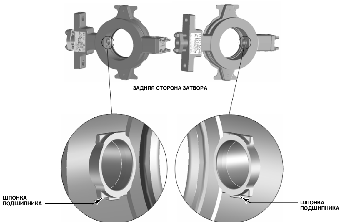
Рис. 6. Положение шпонок подшипника
