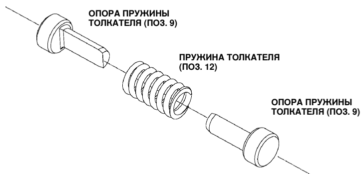
Рис. 9. Узел пружины толкателя и опоры пружины
