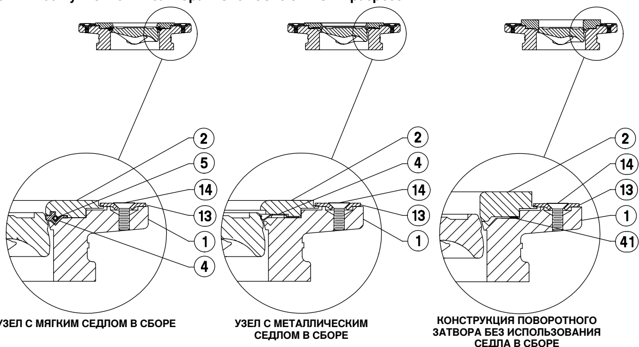
Рис. 12. Узел уплотнения затвора Fisher Control-Disk в разрезе
