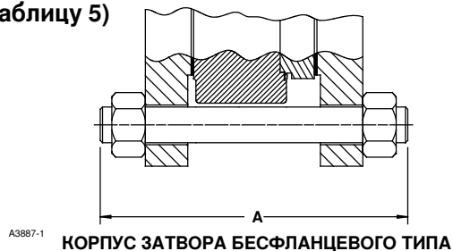
Рис. 3. Резьбовые шпильки для установки (также см. таблицу 5)
