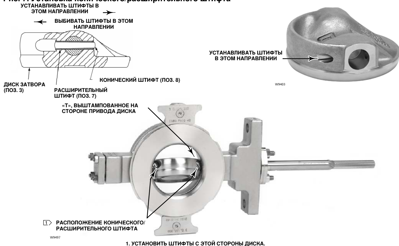
Рис. 7. Установка конического/расширительного штифта
